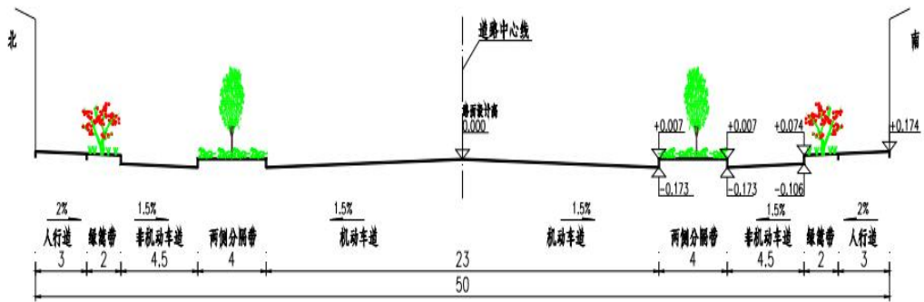
图 2 城市主干路横断面图（50m）
